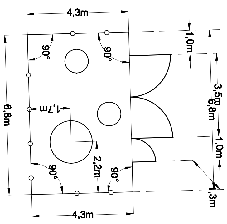
Wymiary ogrodzenia
